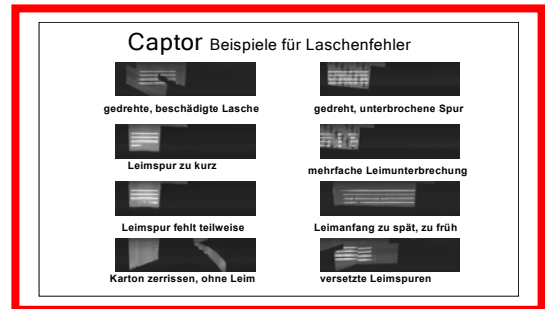
visuelle Leimfehler im Jobspeicher für QS- Nachkontrolle, Abspeicherung
